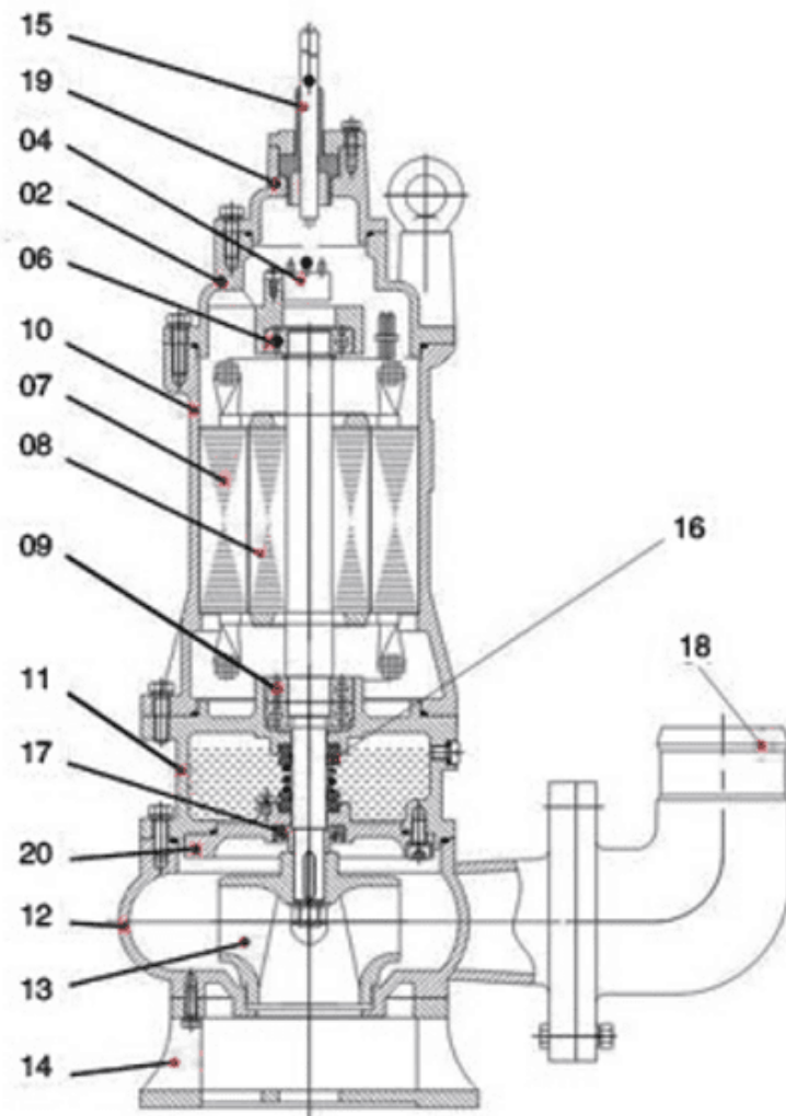
WQ(D) 0.75 - 7.5 kW
