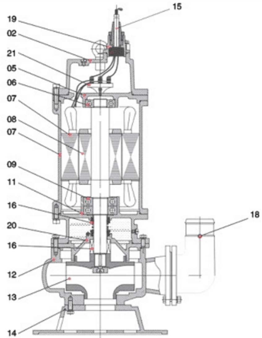
WQ 11 - 45 kW
